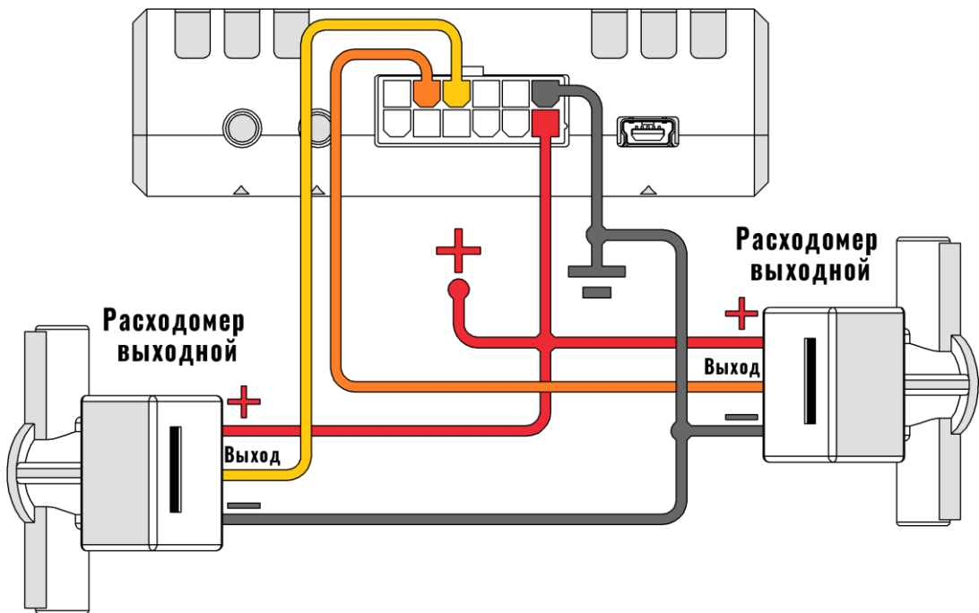
Рисунок 2.13 Пример подключения расходомеров в дифференциальном режиме
