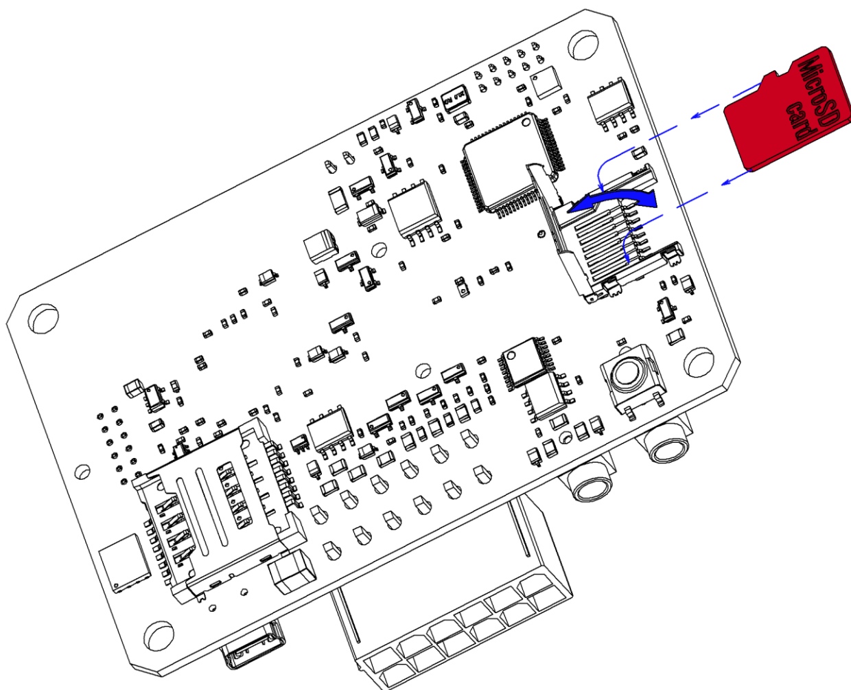
Рисунок 2.6 Установка microSD-карты
