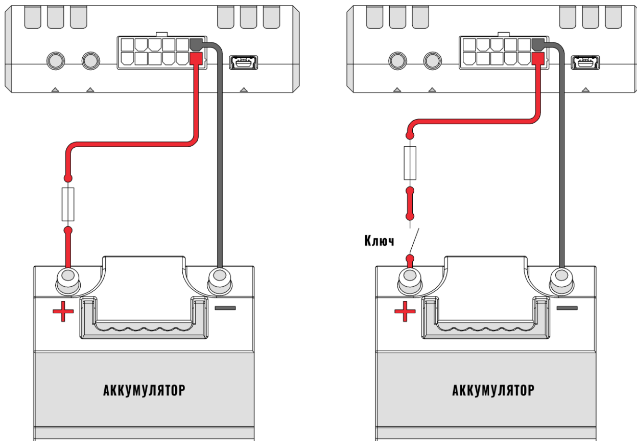
Рисунок 2.7 Подключение питания
