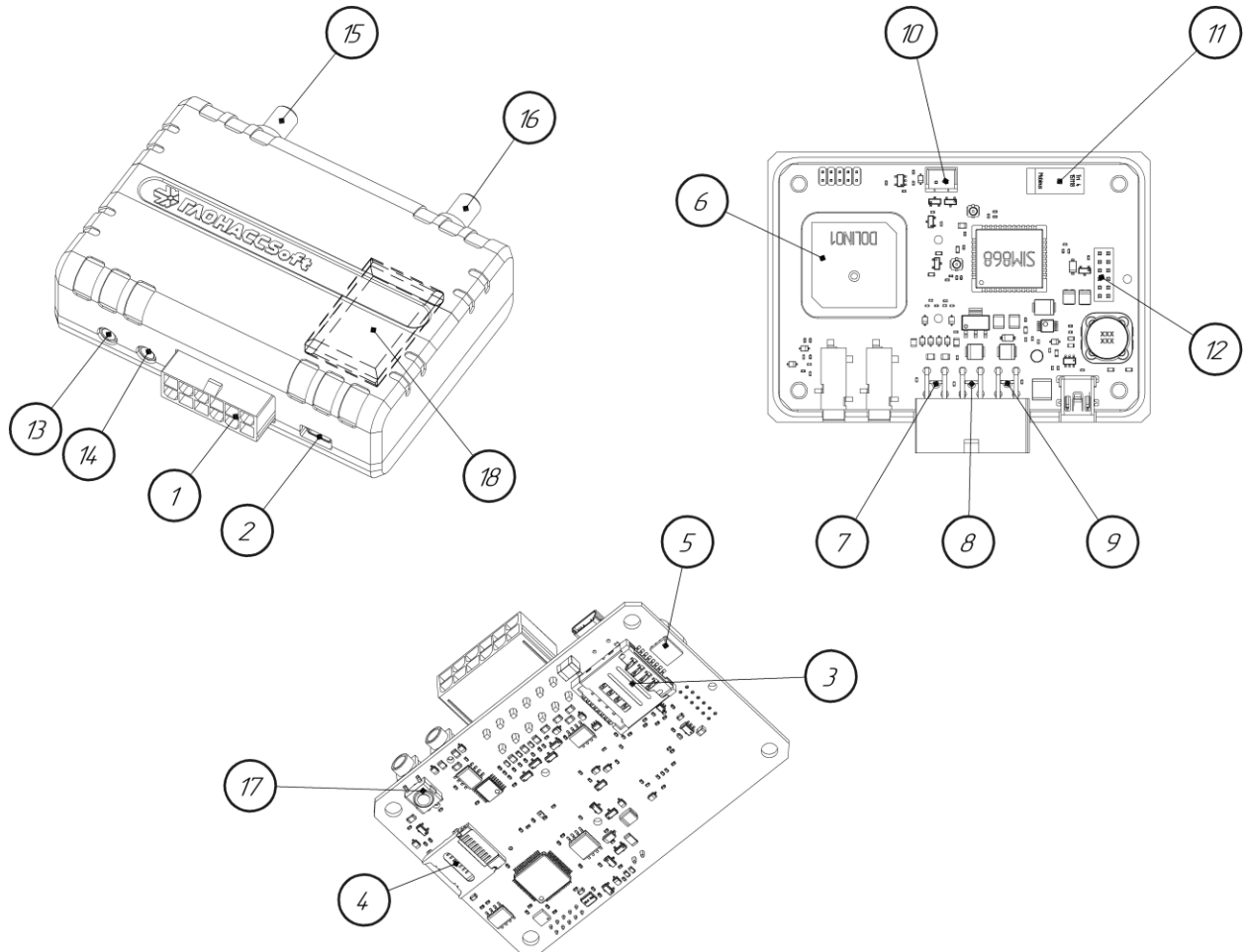
Рисунок 2.1 Основные элементы терминала
